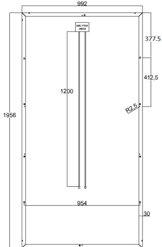
裏面図
